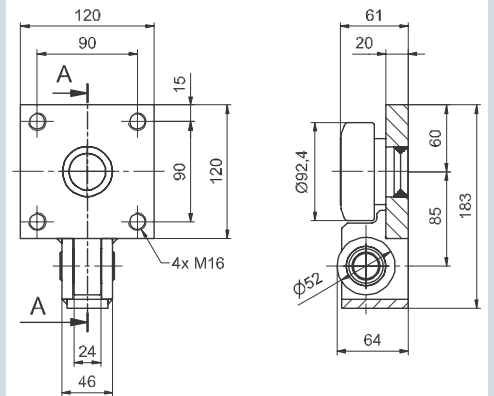
Rolle / Roller XSTR 090.6200
